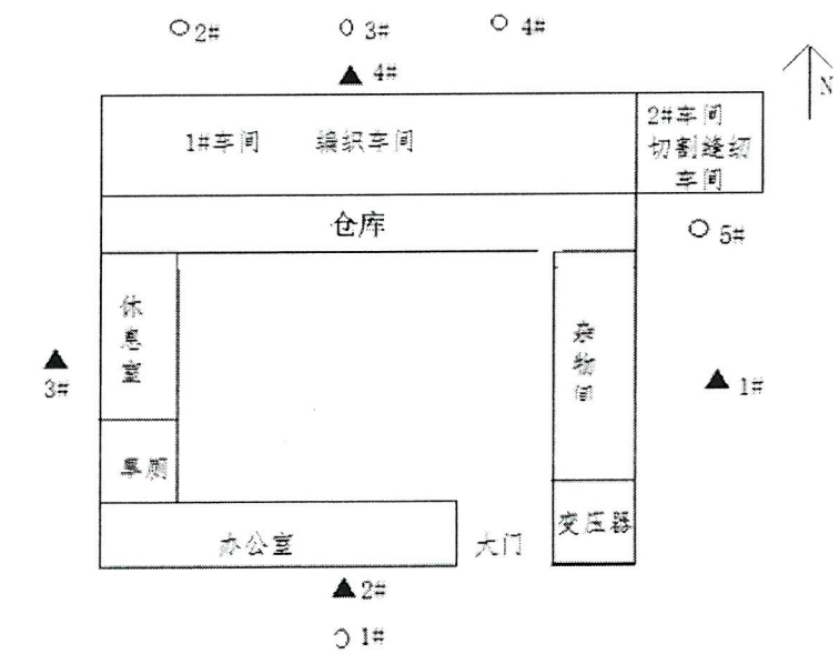
厂界无组织、噪声监测点位示意图
