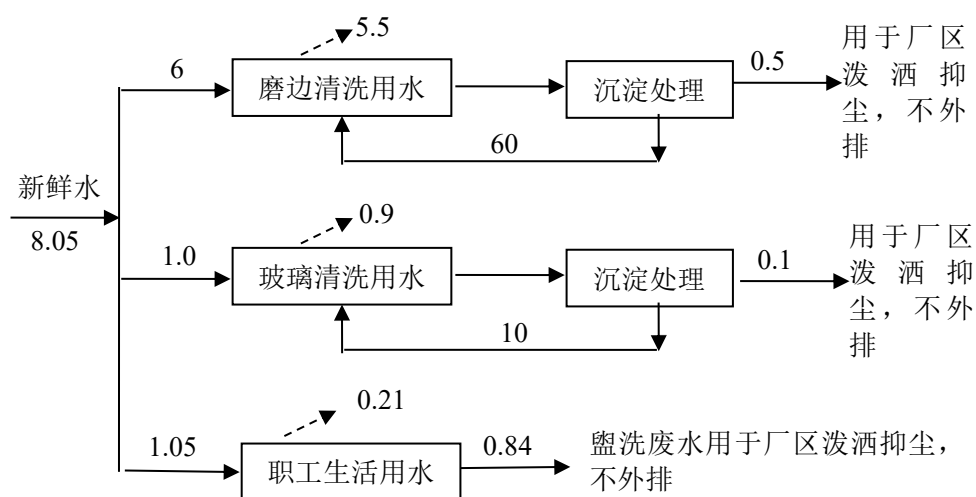
图 2-1 改建项目完成后全厂水平衡图（单位：m³/d）
